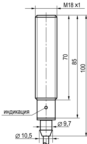
Габаритный чертёж
